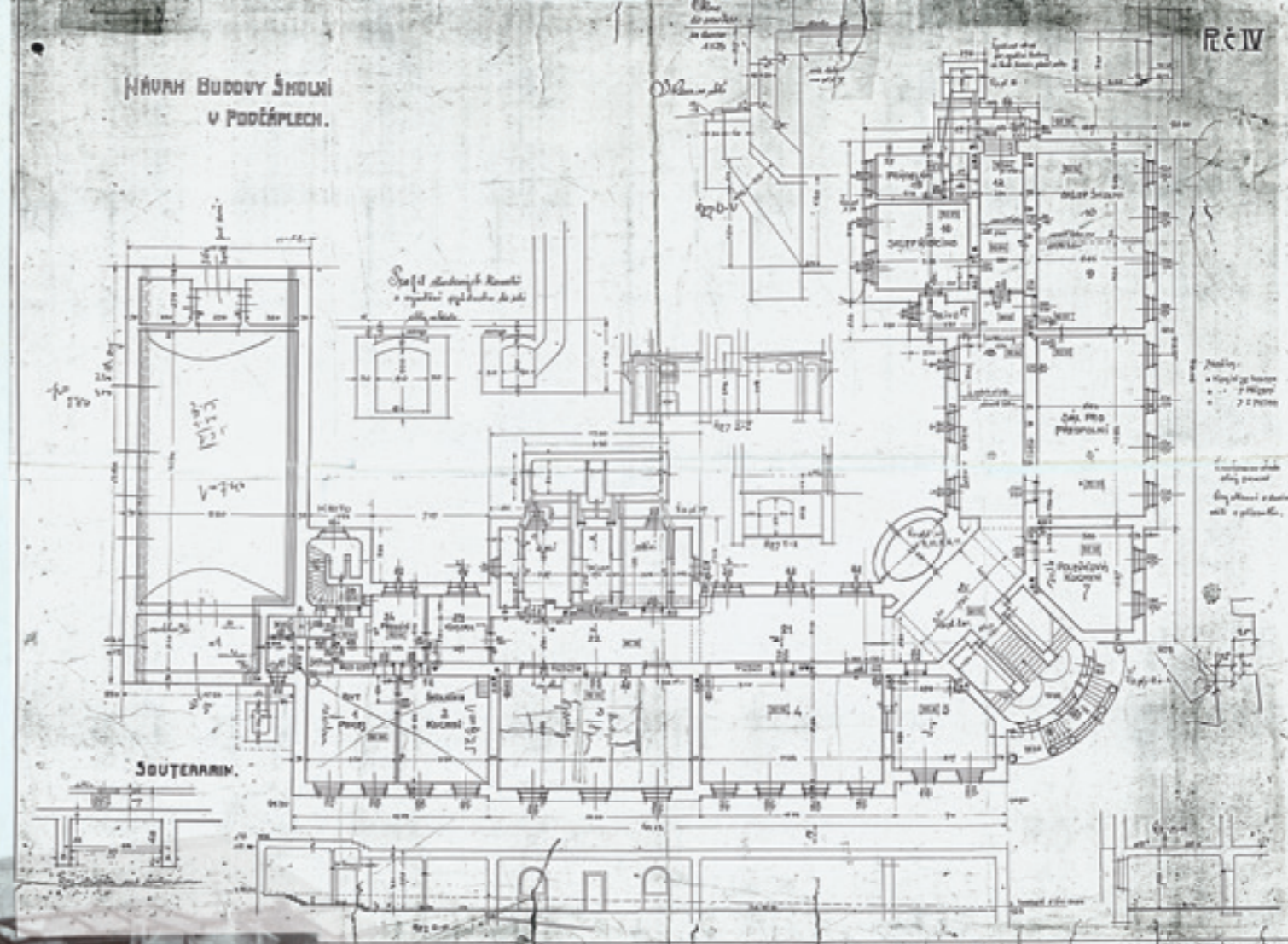
Půdorys Valečkova návrhu
